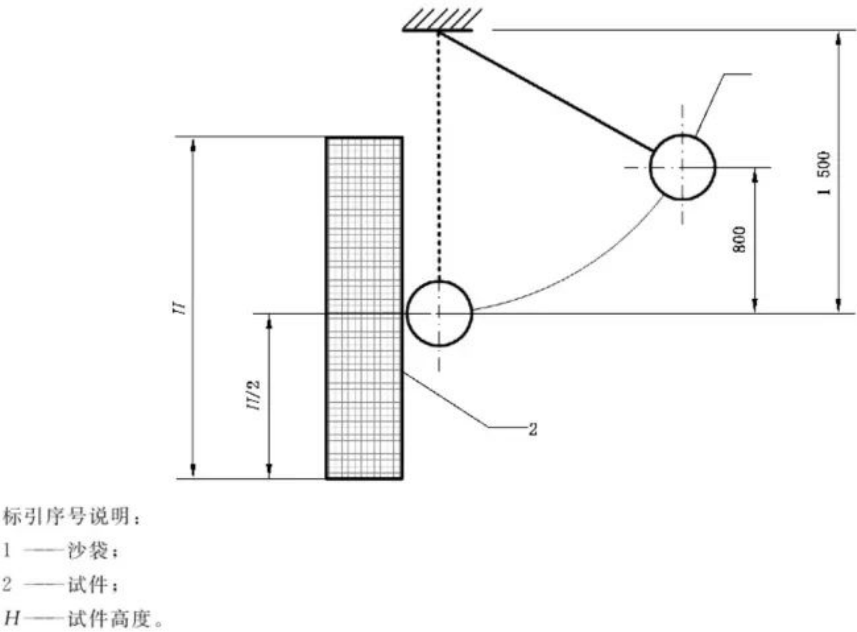
图 2 防闯入性能试验
