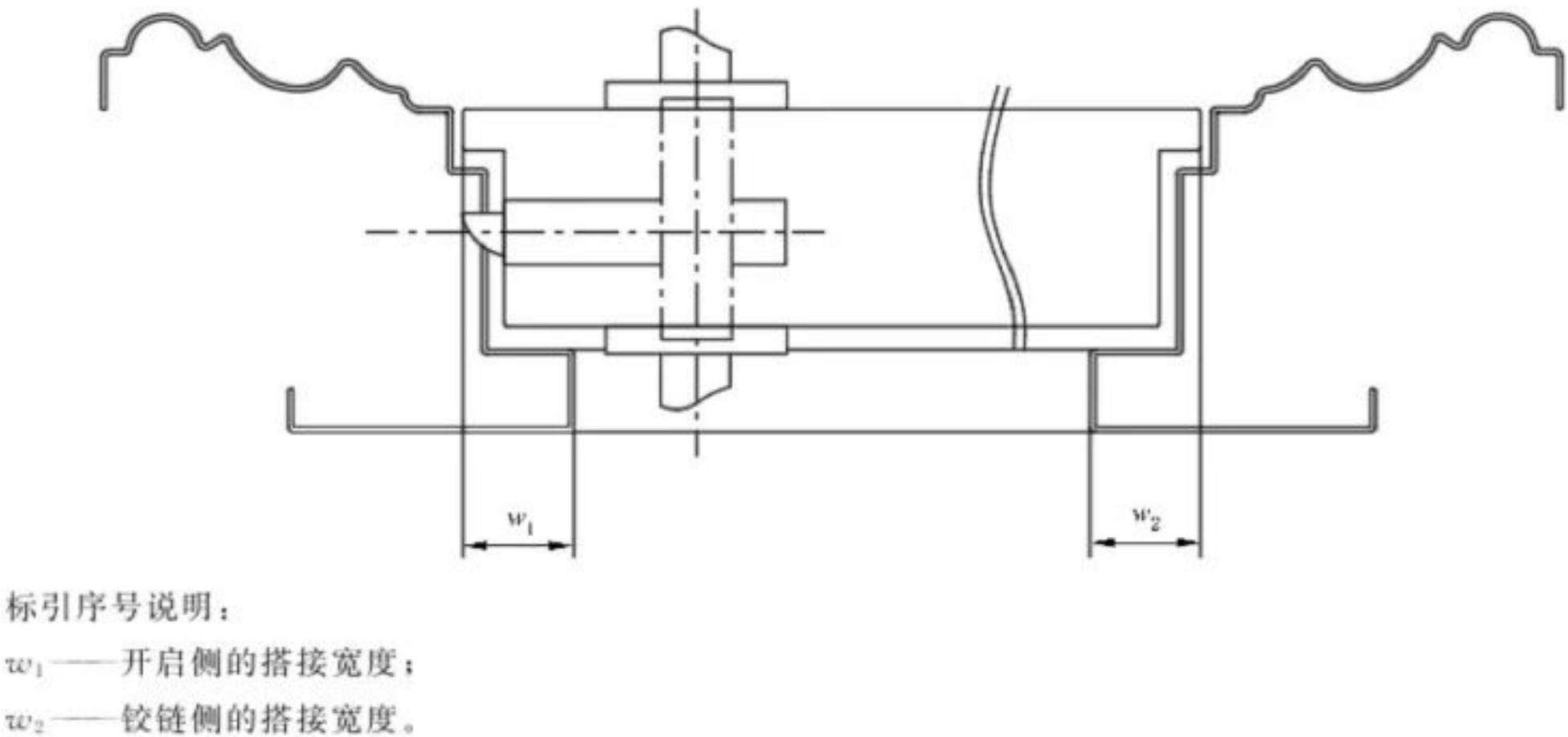
图 1 框扇搭接宽度示意图
